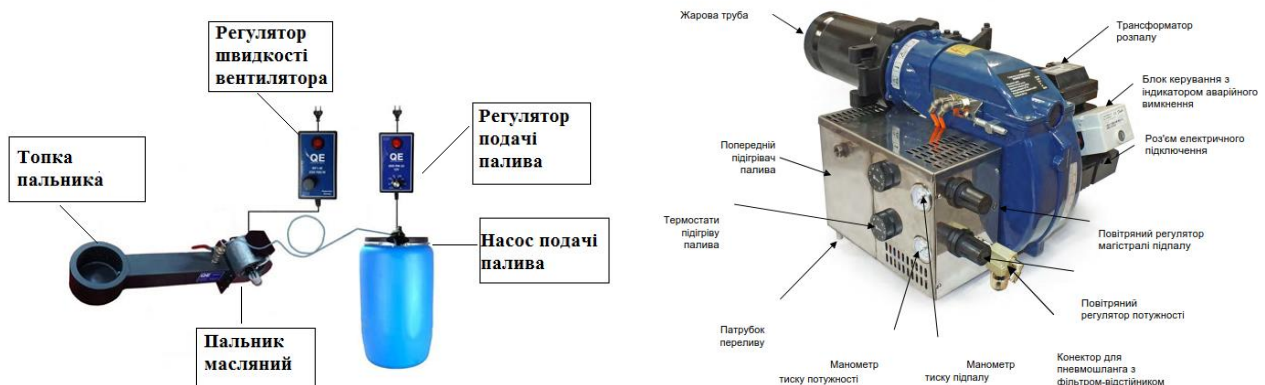
Рис.4 Будова комплекту масляного пального до котла «Retra-Heat»
