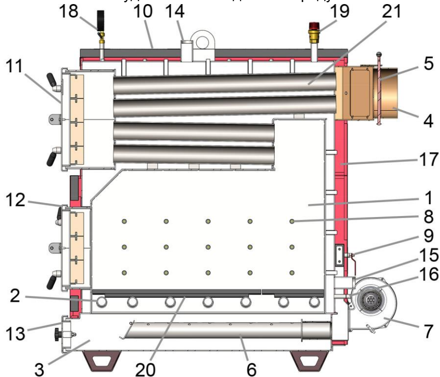
Рис.2 Схема будови котлів модельного ряду «Retra-Heat»
