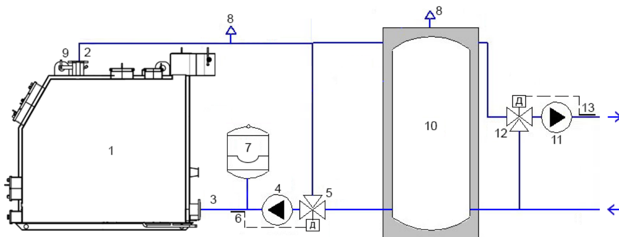
Рис.6 Схема об'язки котла з баком акумулятором (рекомендована)
