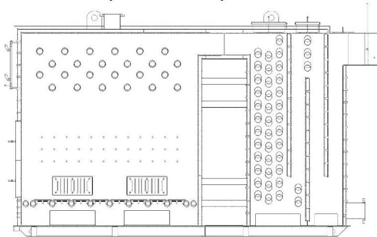
Рис.3д Будова котлів потужністю 2000кВт:
