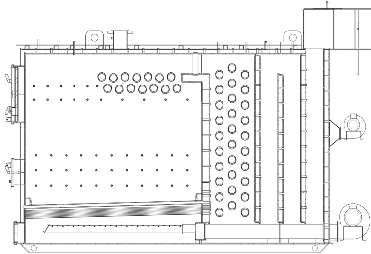
Рис.3г Будова котлів потужністю 1500кВт:
