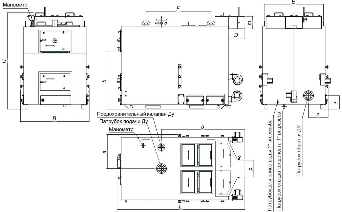
Рис.1 Габаритні і приєднувальні розміри котлів модельного ряду «Retra-3M» потужністю 250-350 кВт
