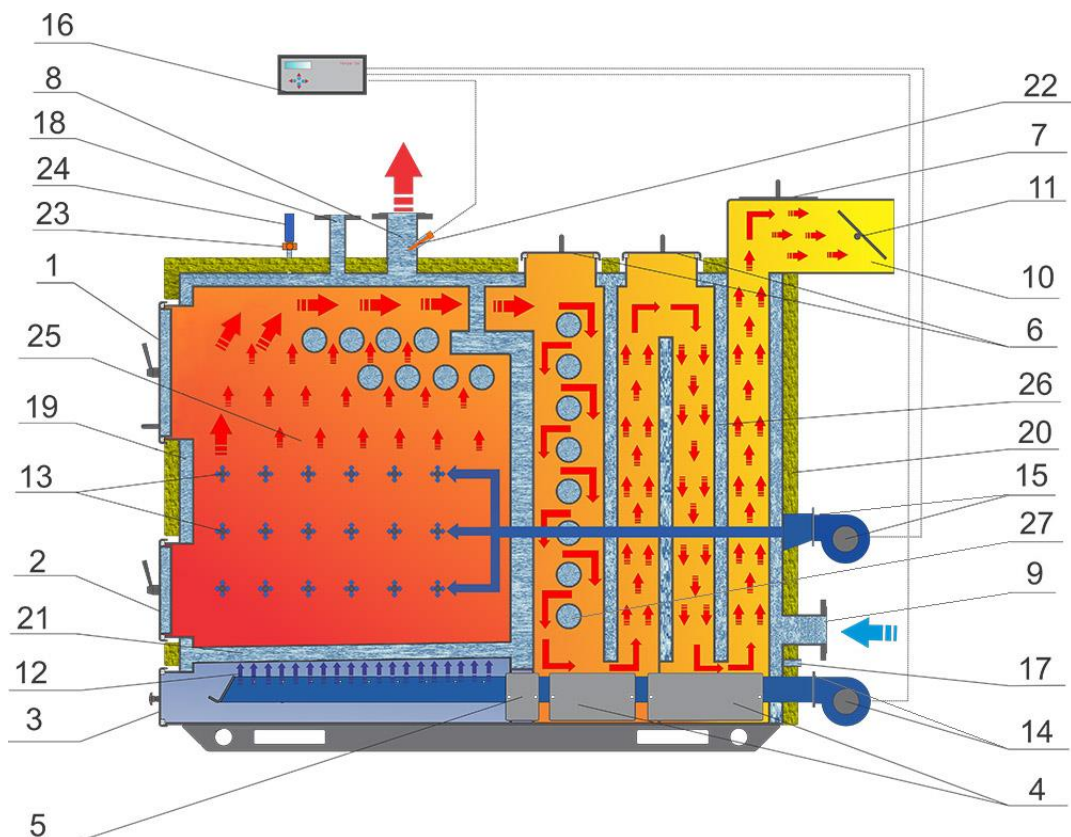
Рис.3 Будова котлів модельного ряду «Retra-3M» потужністю 250-2000кВт
