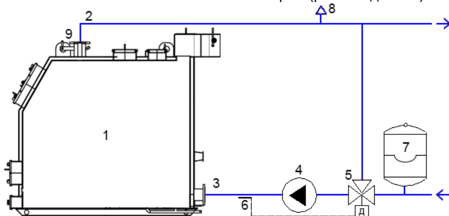
Рис.7 Схема обв'язки котла з бойлером (рекомендована)
