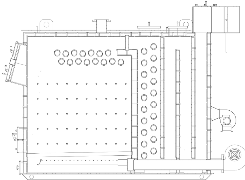
Рис.3в Будова котлів потужністю 1250кВт :
