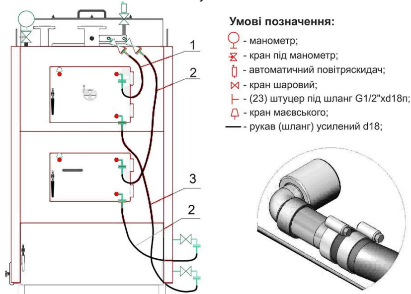
Рис.8 Схема під'єднання рукавів водоохолодження люків для котлів модельного ряду «Retra-3M» потужністю 250-350кВт
