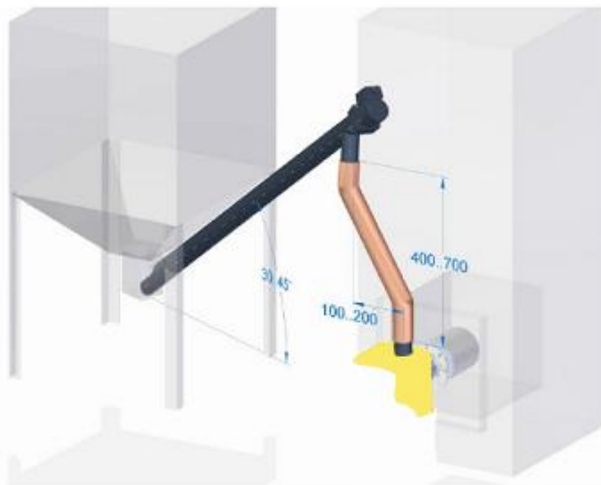
Рис.7- Требования к установке шнека бункера
