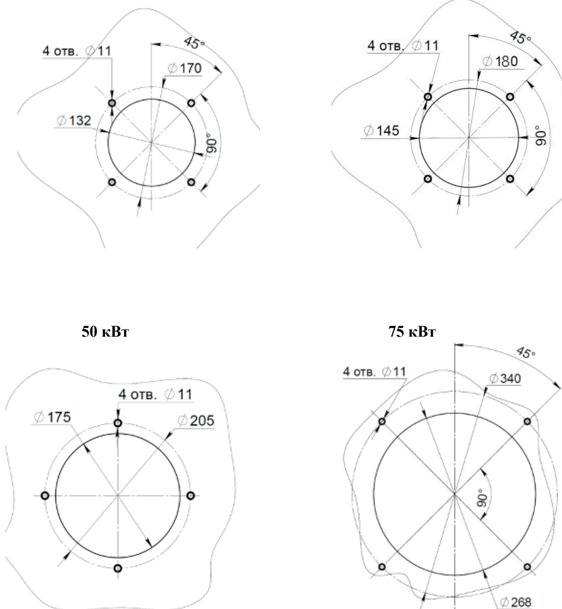
Рисунок 6 – Монтажные отверстия в дверце котла
