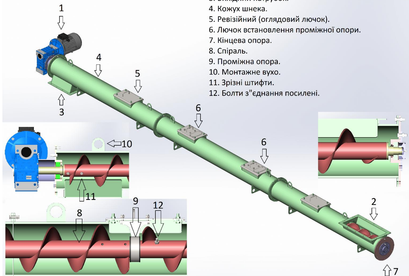
Будова шнекового транспортера ШК-7,3.
